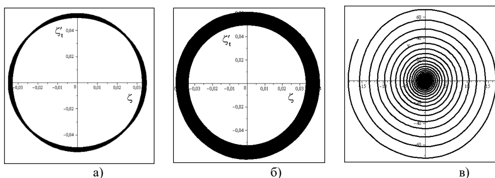
Рис.2. Фазові портрети
