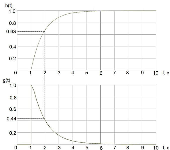
Рис. 3. Визначення сталої часу для об'єкта 1-го порядку по перехідній та імпульсній характеристикам.
