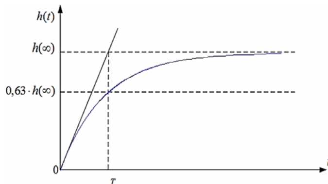
Рис. 1. Графічне визначення сталої часу інерційної ланки першого порядку.
