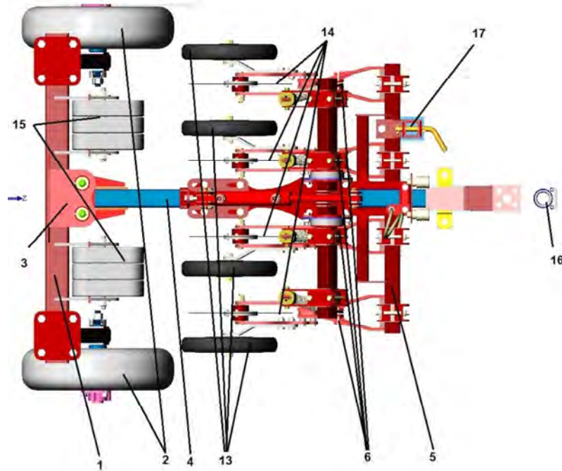
Рис. 15. Загальний вигляд інформаційно-технічної системи оперативного моніторингу агробіологічного стану ґрунтового середовища сільськогосподарських угідь конструкції Олександра Броварця (вид зверху).
