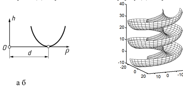
Рис. 2. Схема утворення поверхні за заданою кривою осьового перерізу: а) розташування кривої в плоскій системі координат; б) поверхня, утворена гвинтовим рухом заданої кривої
