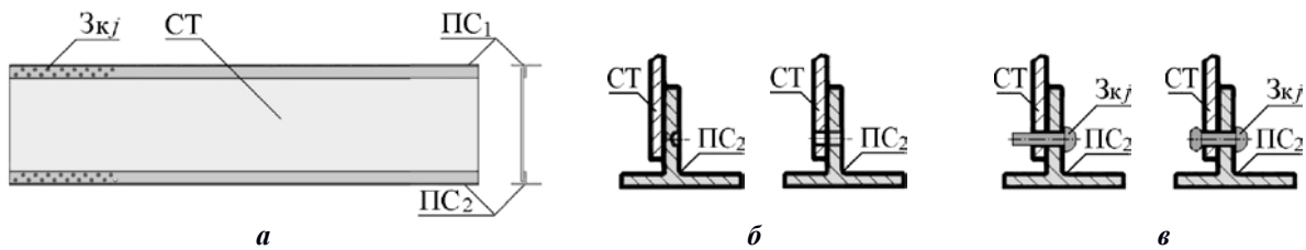
Рис. 3. Клепаання поясів PC_1 і PC_2 до стінки СТ лонжерона крила: а – загальний вид; б – початок і завершення свердління отвору; в – початок і завершення клепаання заклепки Зк_j
