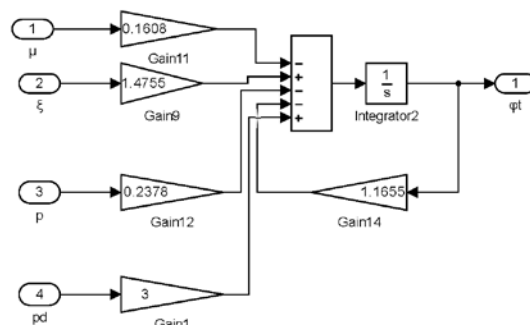
г) Модель гібридного турбокомпресора
