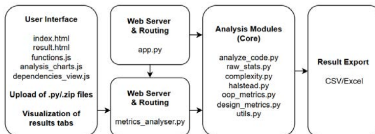
Рис. 1. Архітектура програмної системи статичного аналізу коду Code Analyzer
