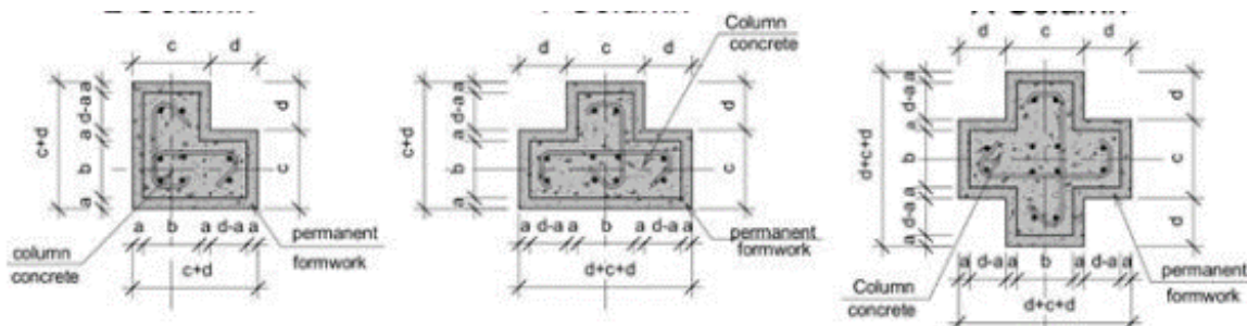
Рис. 8. Пропонована та використана конфігурація колон і балок
