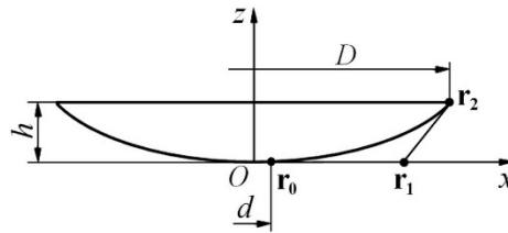
Рис. 1. Схема побудови узагальненої геометричної моделі робочих поверхонь ґрунтообробних дисків:
