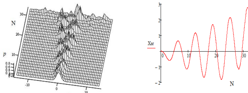
Рис. 5. Еволюція щільності пакета і центру пакету X_{sr} розподілу ймовірностей p(x,t) ; g = 0.2 , \sigma_w = 1.2
