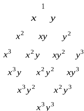
Рис. 2. Схема Паскаля. Бікубічний елемент Лагранжа
