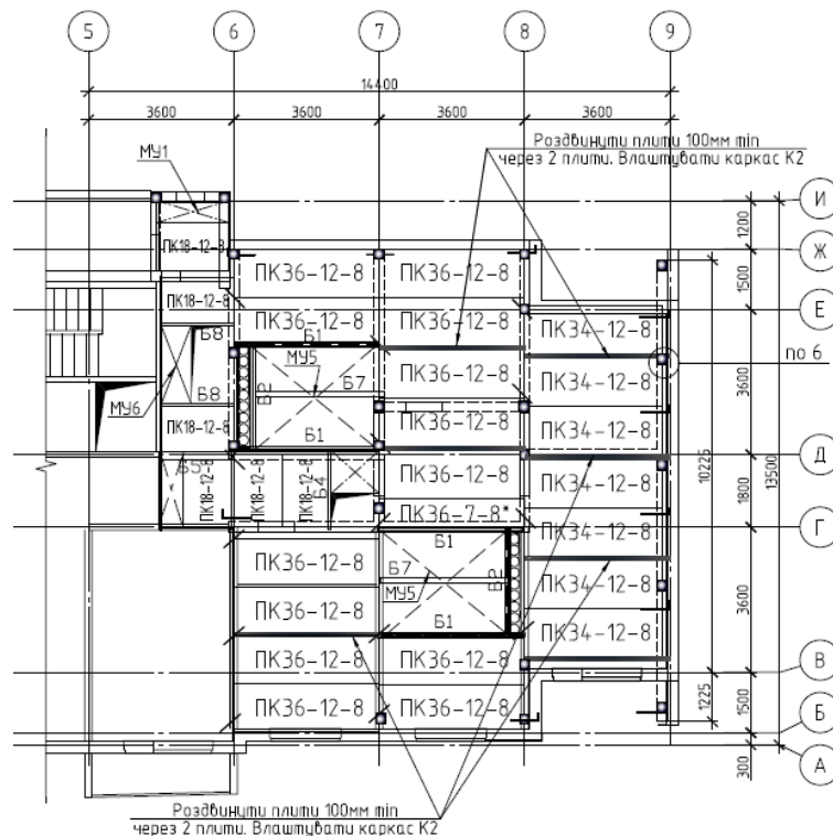
Рис. 9. Влаштування збірних перекриттів
