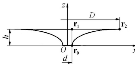
Рис. 2. Модифікація схеми формування поверхні диска
