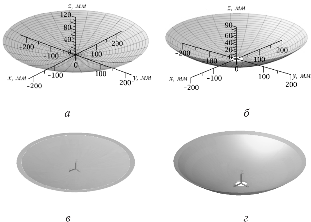
Рис. 6. Сферичні та торові ґрунтообробні знаряддя: а – D=450 мм, R=600 мм; б – D=400 мм, R=300 мм, d=40 мм; в – D=350 мм, R=600 мм, \delta=5 мм; г – D=400 мм, R=300 мм, d=30 мм, \delta=4 мм
