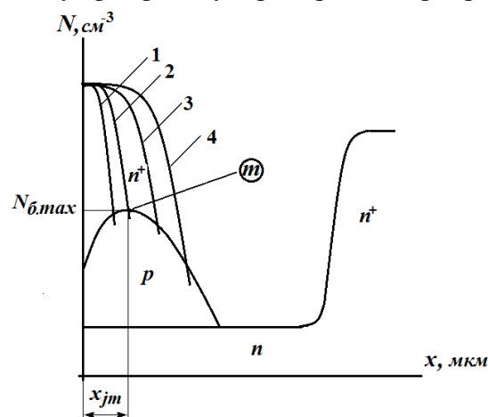
Рис. 3. Реальний розподіл домішок у дрейфовому п-р-п-транзисторі
