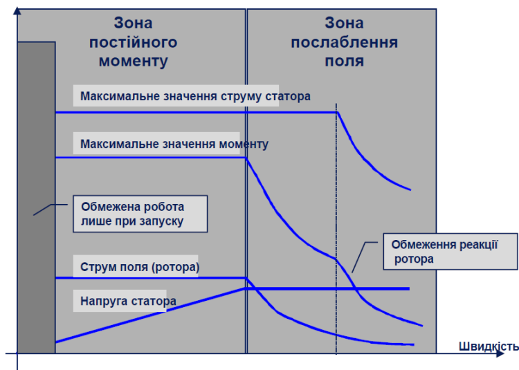
Рис. 4. Характеристики меж експлуатації для синхронного двигуна з перетворювачем інверторного типу з джерелом струму
