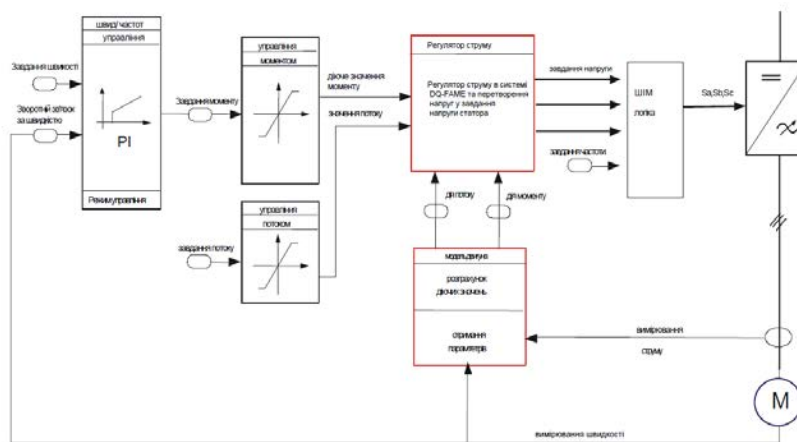
Рис. 7. Функціональна схема роторного векторного управління
