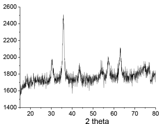
Рис. 1. Дифрактограма магнетиту
