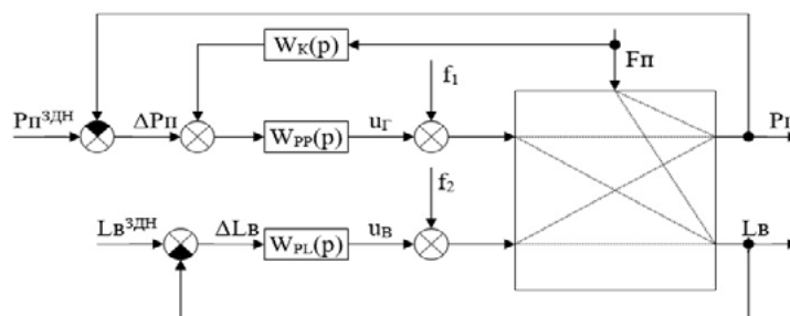
P_n^{зад} , L_v^{зад} – задані значення тиску гріючої пари та рівня води в барабані котла; \Delta P_n , \Delta L_v – помилки регулювання тиску гріючої пари та рівня води в барабані; W_K(p) , W_{PP}(p) , W_{PL}(p) – передаточні функції корегуючого зв’язку, регулятора тиску гріючої пари, регулятора рівня води в барабані котла відповідно
