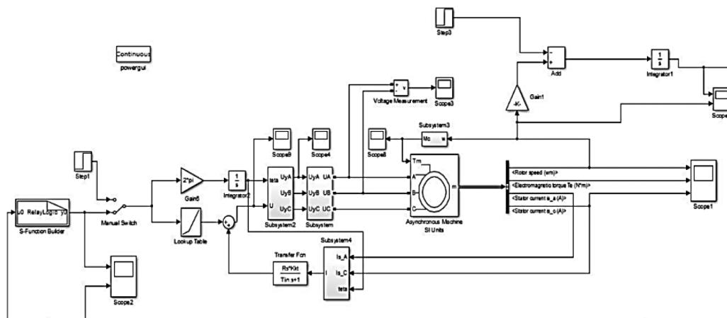
Рис. 5. Імітаційна модель скалярного керування швидкістю обертання АД насосного агрегату з автоматичною системою регулювання води в резервуарі
