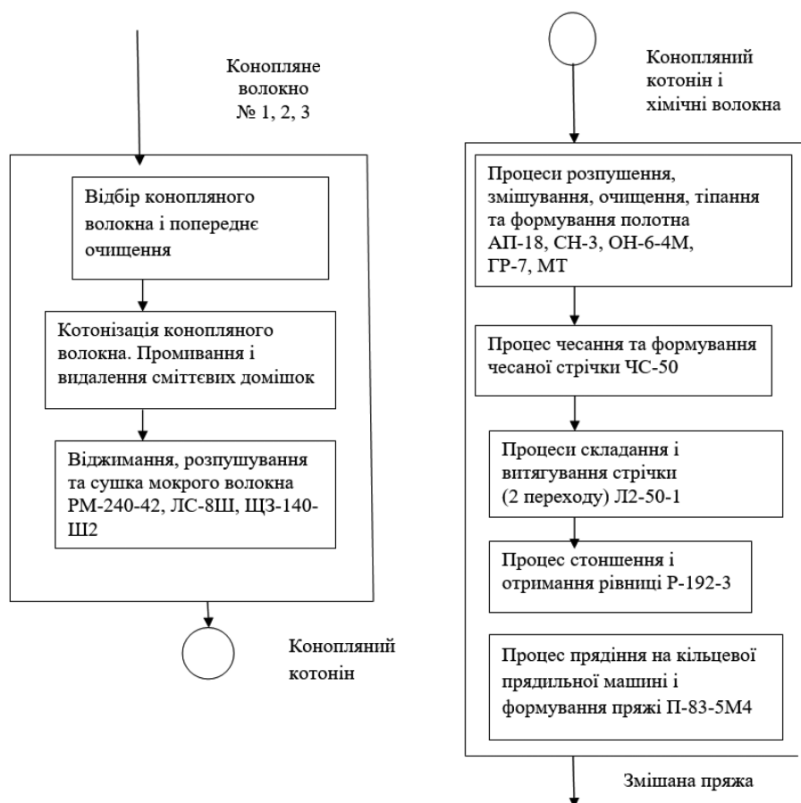
Рис. 2. Схема технологічного процесу отримання багатокомпонентної пряжі з конопляним котоніном
