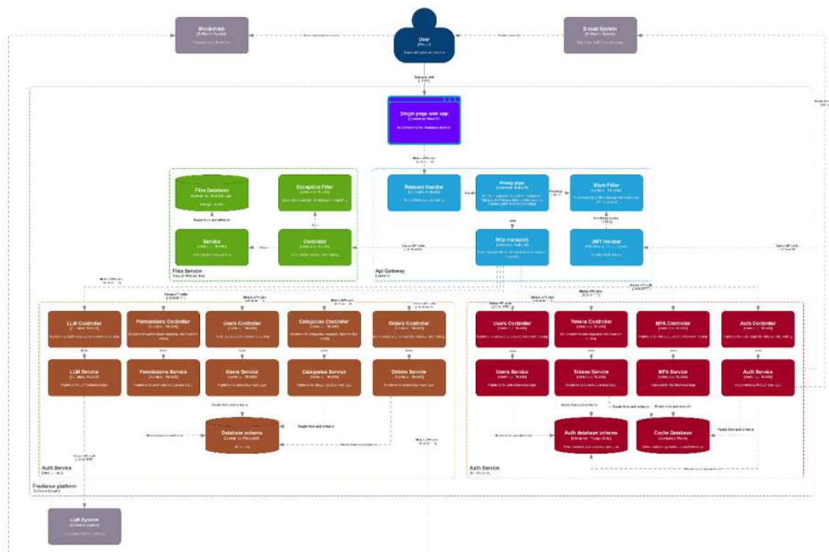
Рис. 3. С4 рівень 3, внутрішня архітектура всіх мікросервісів
